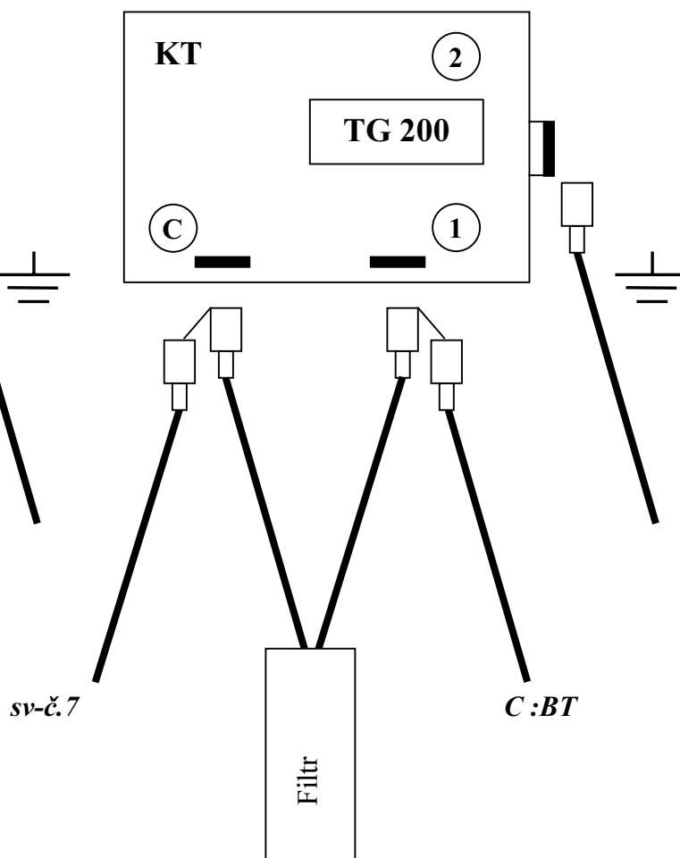
Zapojení se zhášecím členem (filtrem)
